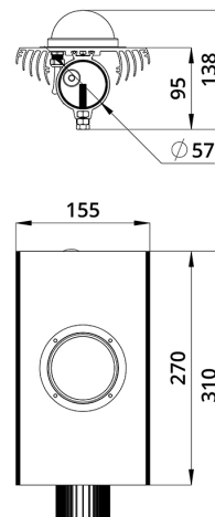
Габаритный чертёж
