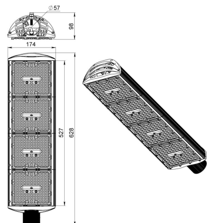
Габаритный чертеж
