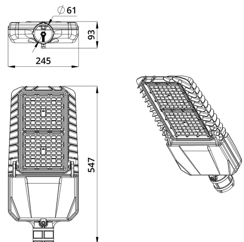
Габаритный чертёж
