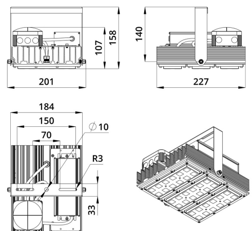
Габаритный чертеж
