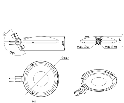
Габаритный чертеж
