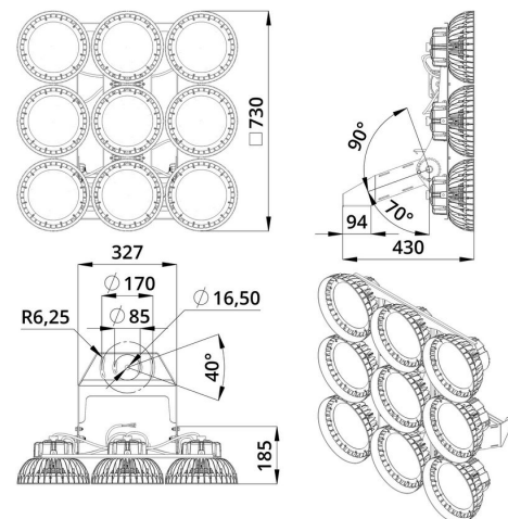
Габаритный чертеж
