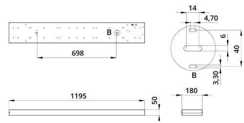
Монтаж светильника
